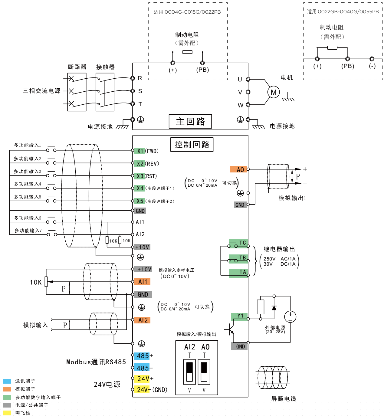
端子配线图
