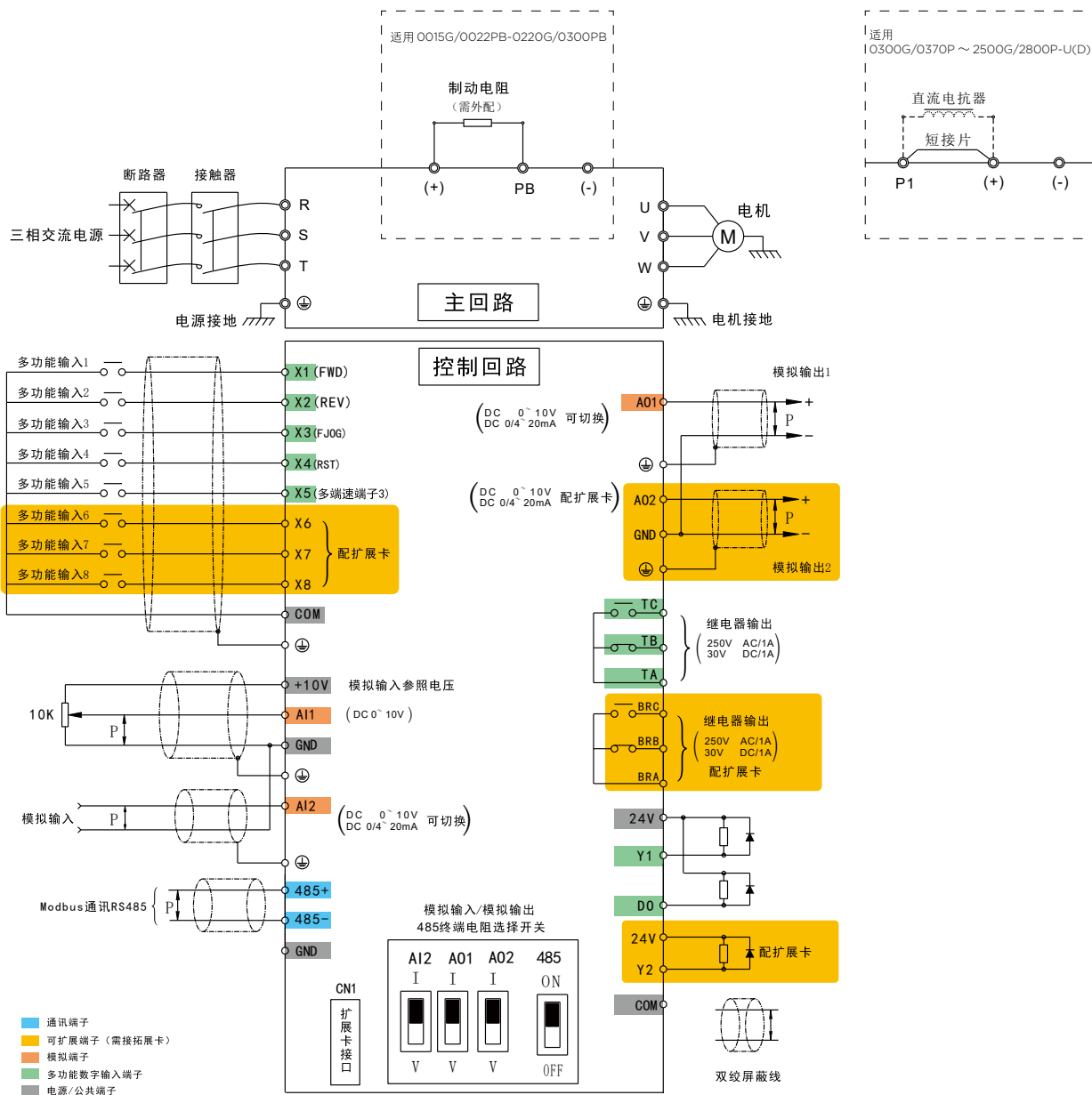
端子配线图
